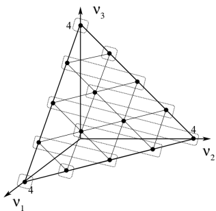
Рис. 1. Классы эквивалентности по правилу Борда
